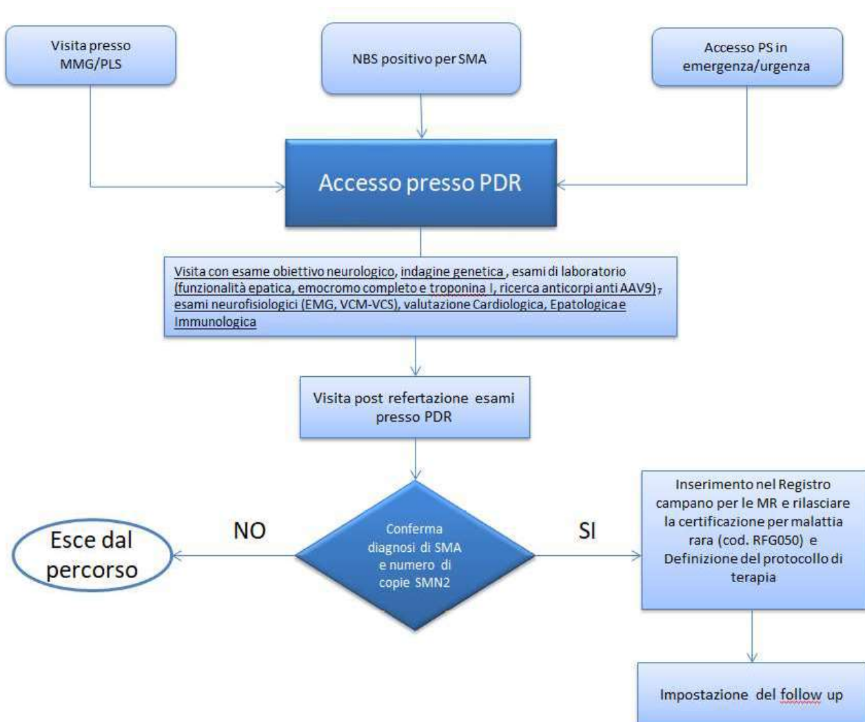
Figura 2: Algoritmo diagnostico
